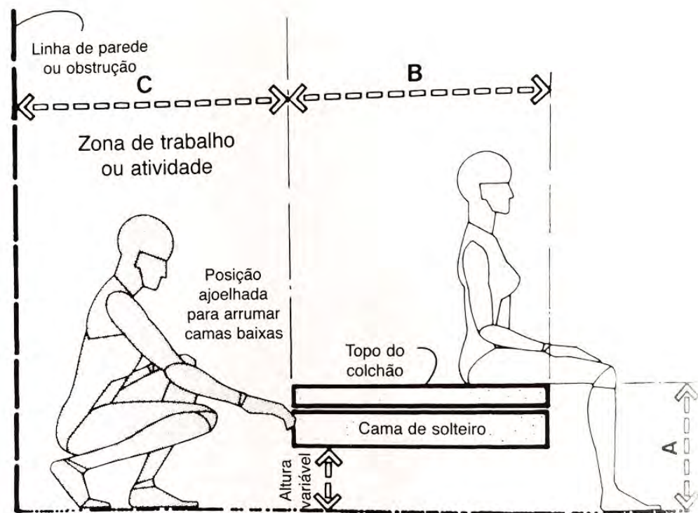
CAMA DE SOLTEIRO / DIMENSÕES E ESPAÇOS LIVRES
