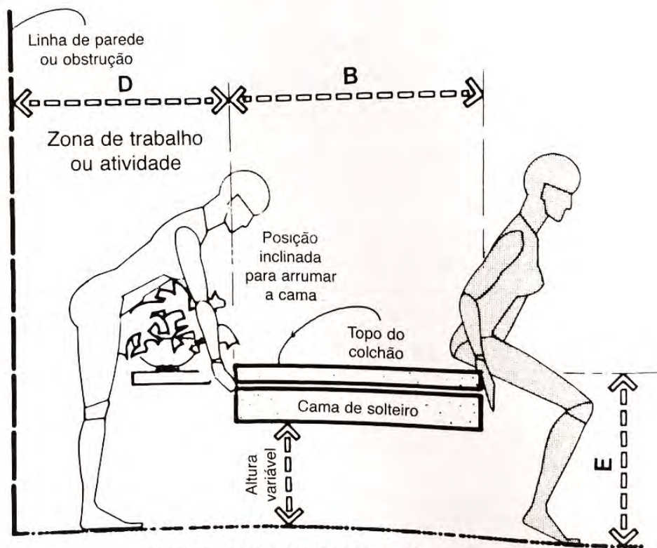
CAMA DE SOLTEIRO / DIMENSÕES E ESPAÇOS LIVRES
