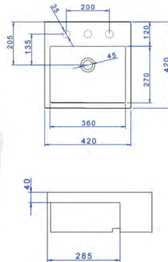
Cuba de Semi-Encaixe Quadrada com Mesa e Porta Toalha Código L.83C Cor Branco 17 ou Ébano 95 Tam.: indicado nos desenhos
